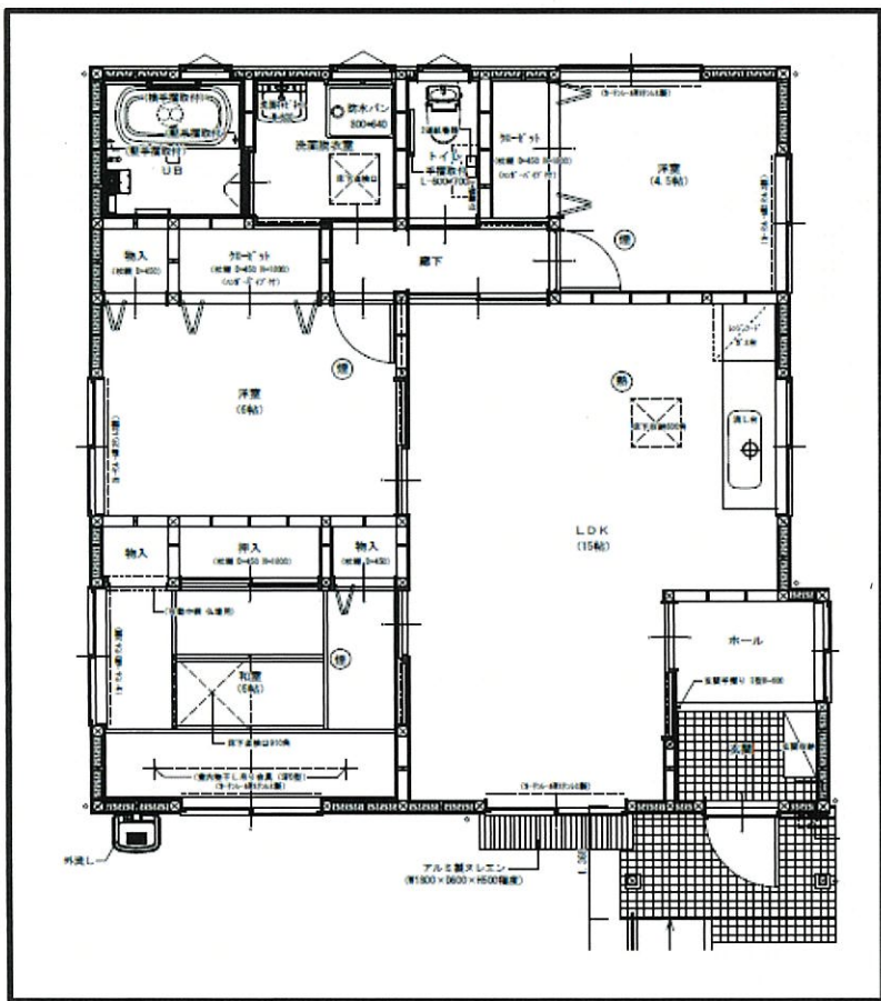
【7. 小野駅前東】3LDK 告知事項有
