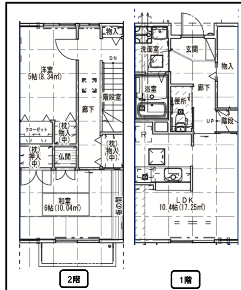
【1. 川前四番】 2LDK
