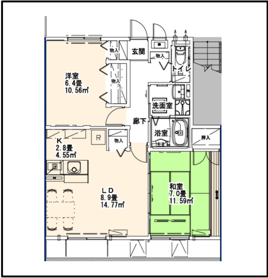
【 13. 小松南 】 2LDK
